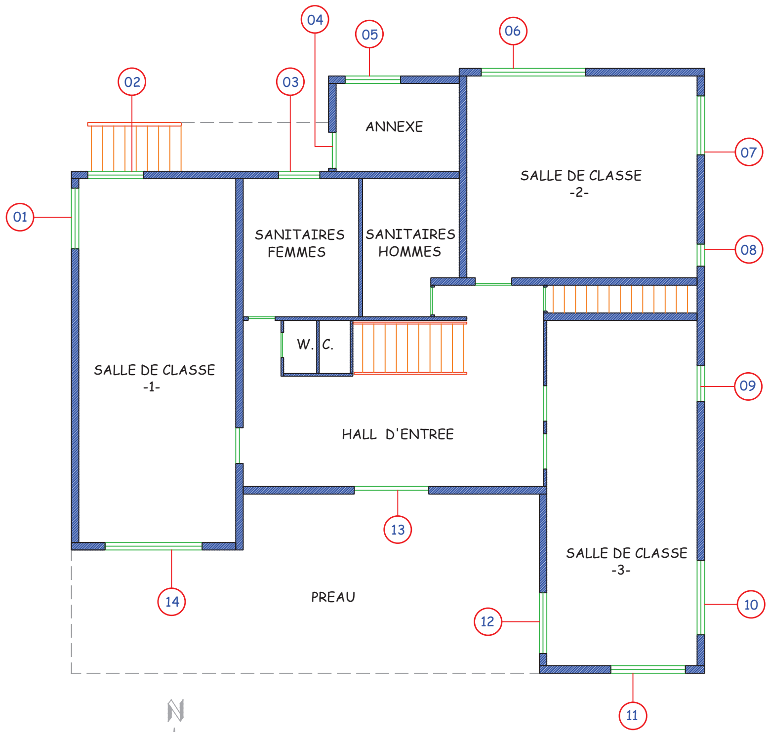
BATIMENT -2- REZ DE CHAUSSEE
